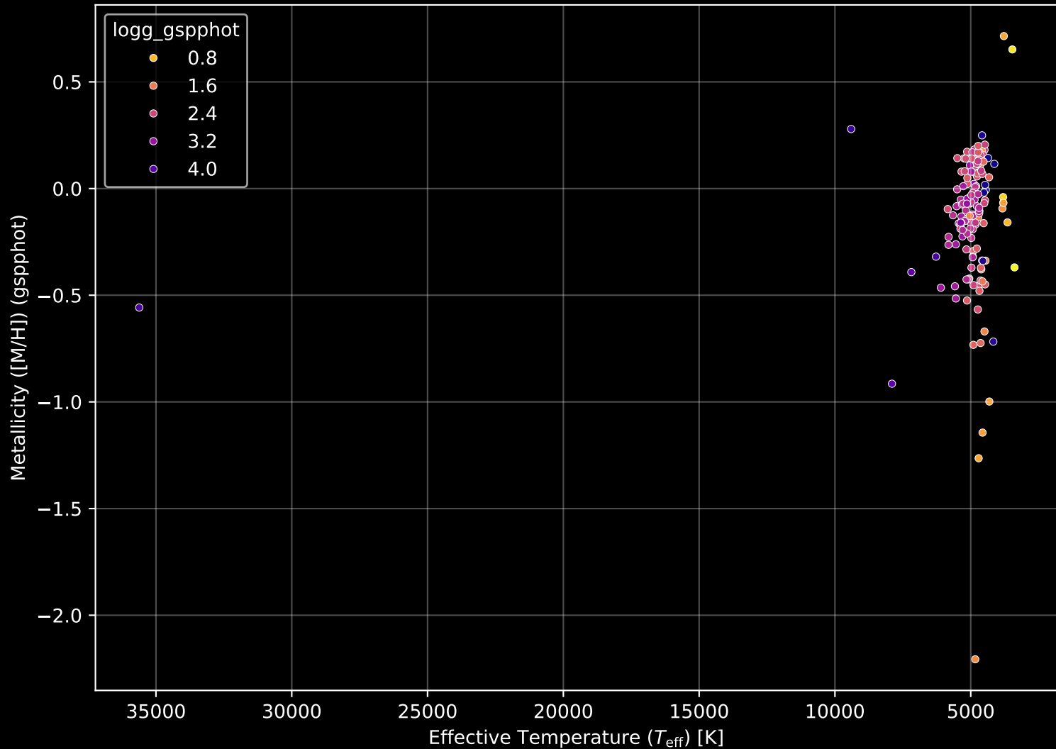
APOGEE DR17 Field: [025+14] Stellar Population Parameters (n= 148)
